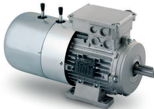
MOTORI AUTOFRENANTI A DOPPIO FRENO E LEVA DI SBLOCCO PER APPLICAZIONI DI SICUREZZA SELF-BRAKING MOTORS WITH DOUBLE BRAKE AND HAND RELEASE FOR SAFETY APPLICATIONS
